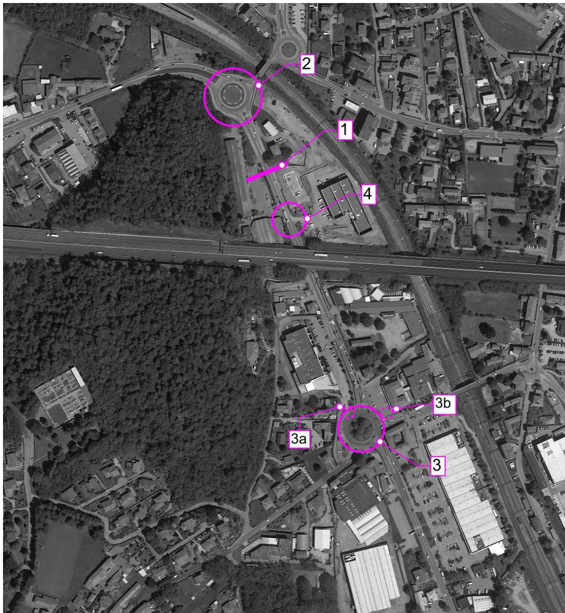
Localizzazione dispositivo radar e conteggio manovre di svolta alle intersezioni
